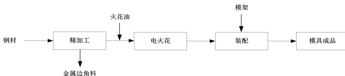
图 5-2 模具生产工艺流程及产污环节节点图
