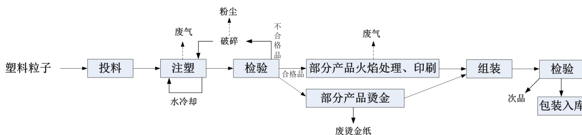
图 5-1 化妆品包装品生产工艺流程及产污环节节点图
